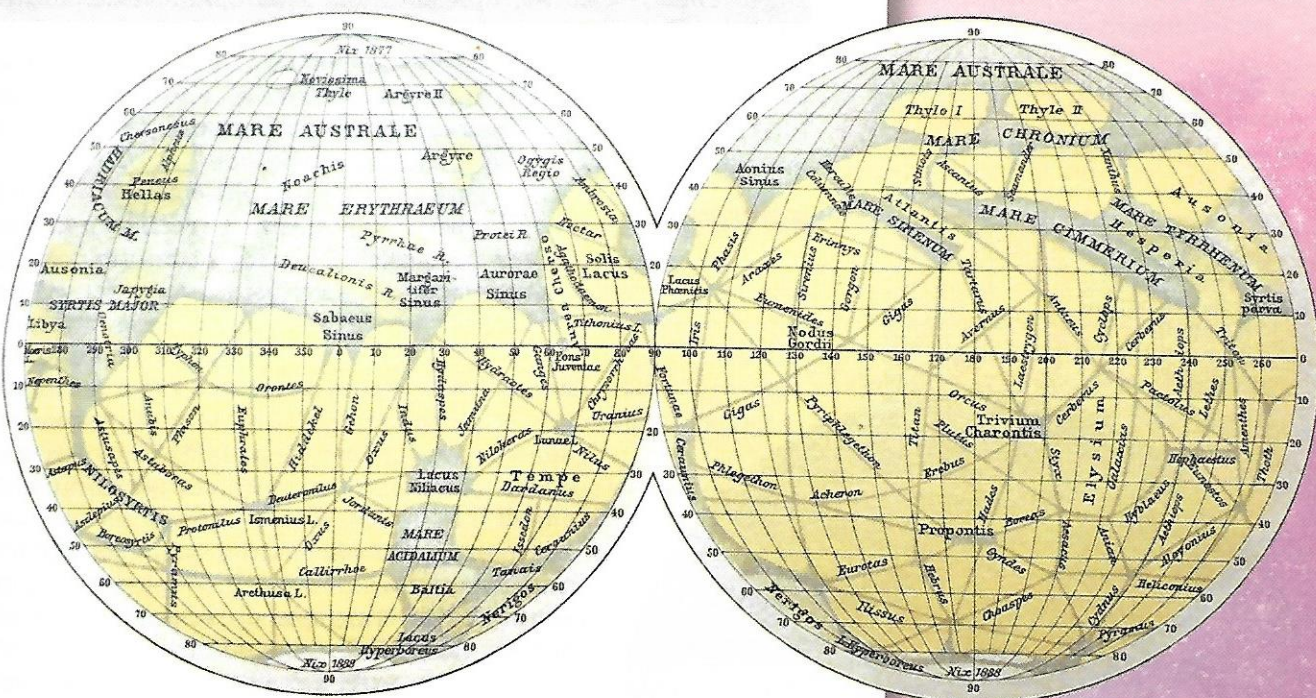
Карта Марса Дж. Скиапарелли
