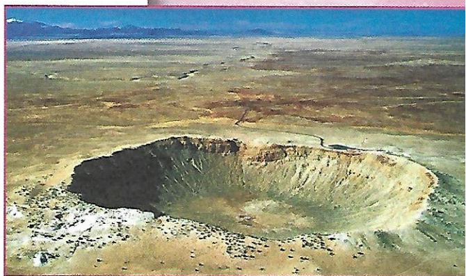
Метеоритный кратер в Аризоне (США)
