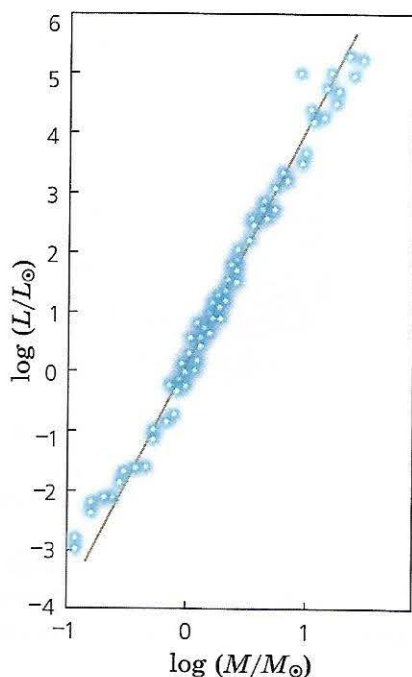
Диаграмма «Масса — светимость» для звёзд главной последовательности
