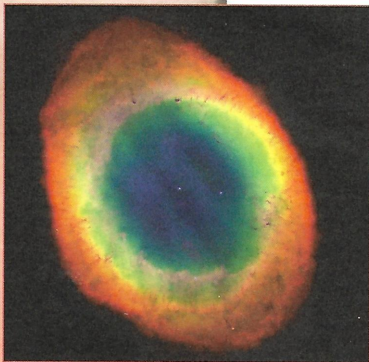
Планетарная туманность «Кольцеобразная» в созвездии Лиры
