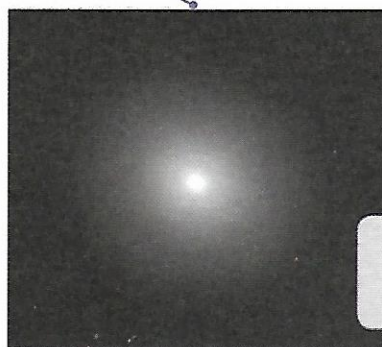
ЭЛЛИПТИЧЕСКАЯ ГАЛАКТИКА
