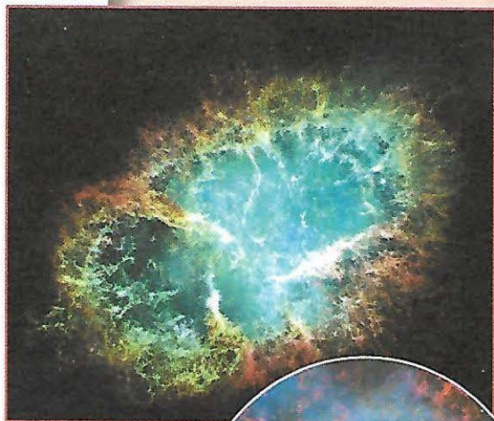
Крабовидная туманность
