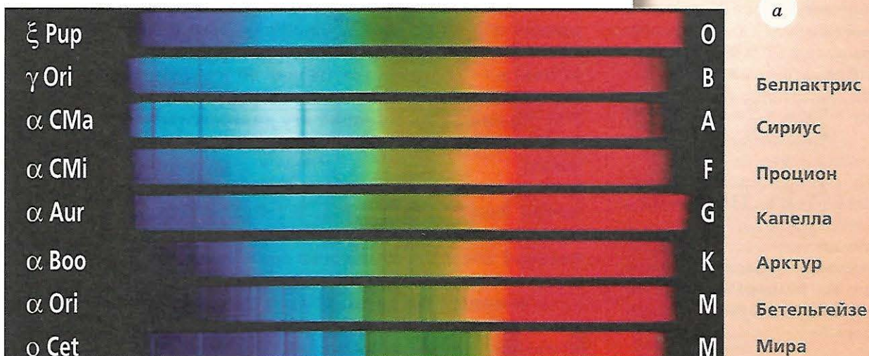
Спектры звёзд различных спектральных классов
