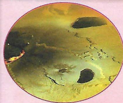
Поверхность спутника Ио
