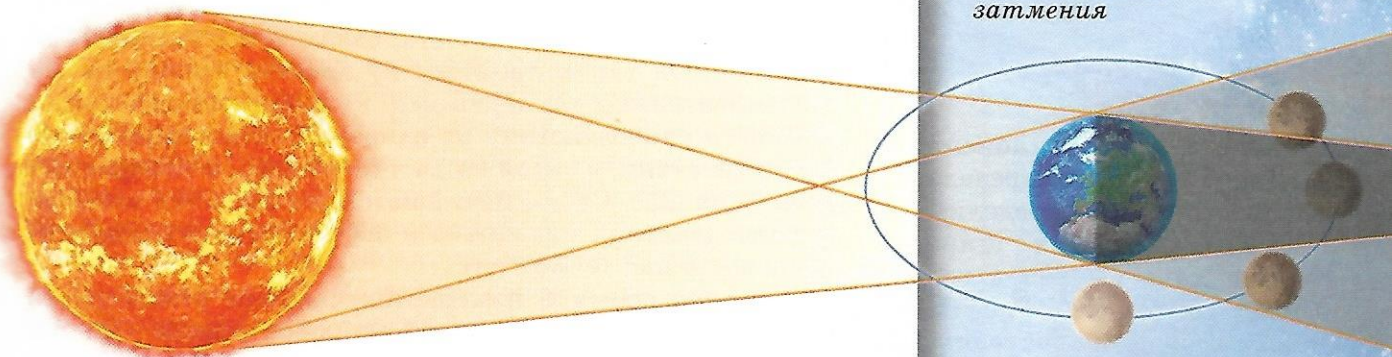
Схема лунного затмения
