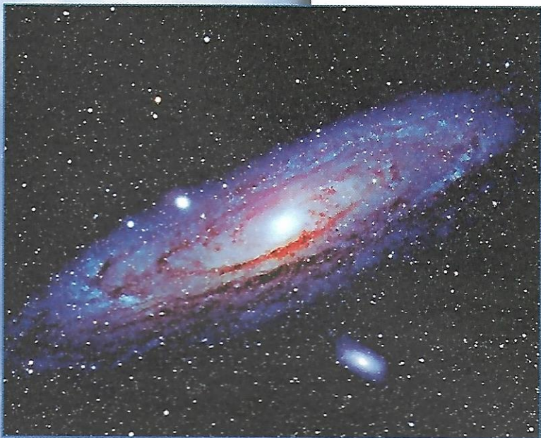
Туманность Андромеды
