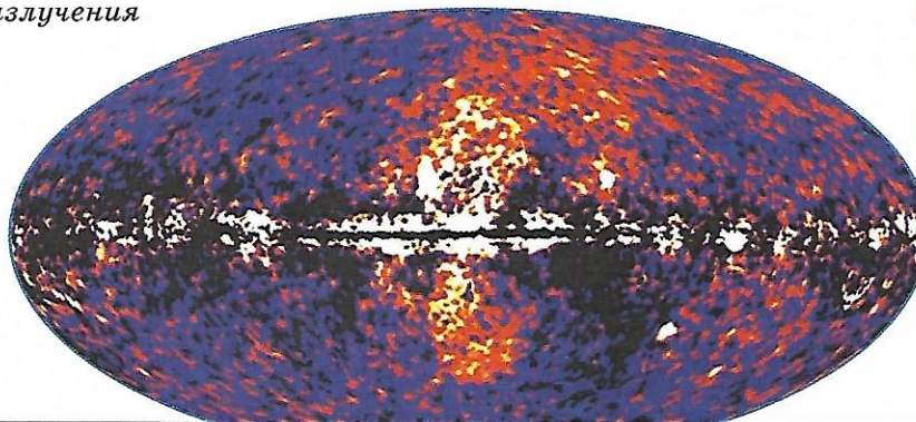
Карта распределения \gamma -излучения
