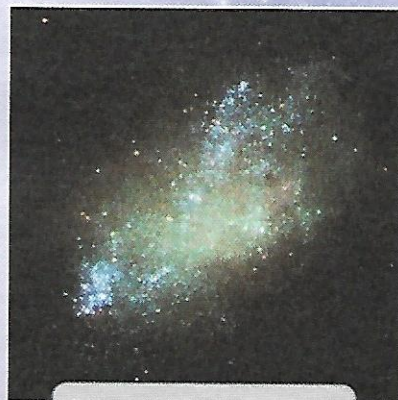
НЕПРАВИЛЬНЫЕ ГАЛАКТИКИ
